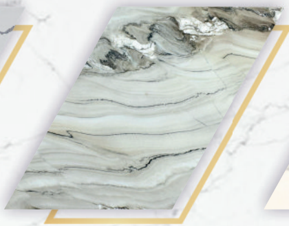
QUARTZITE
